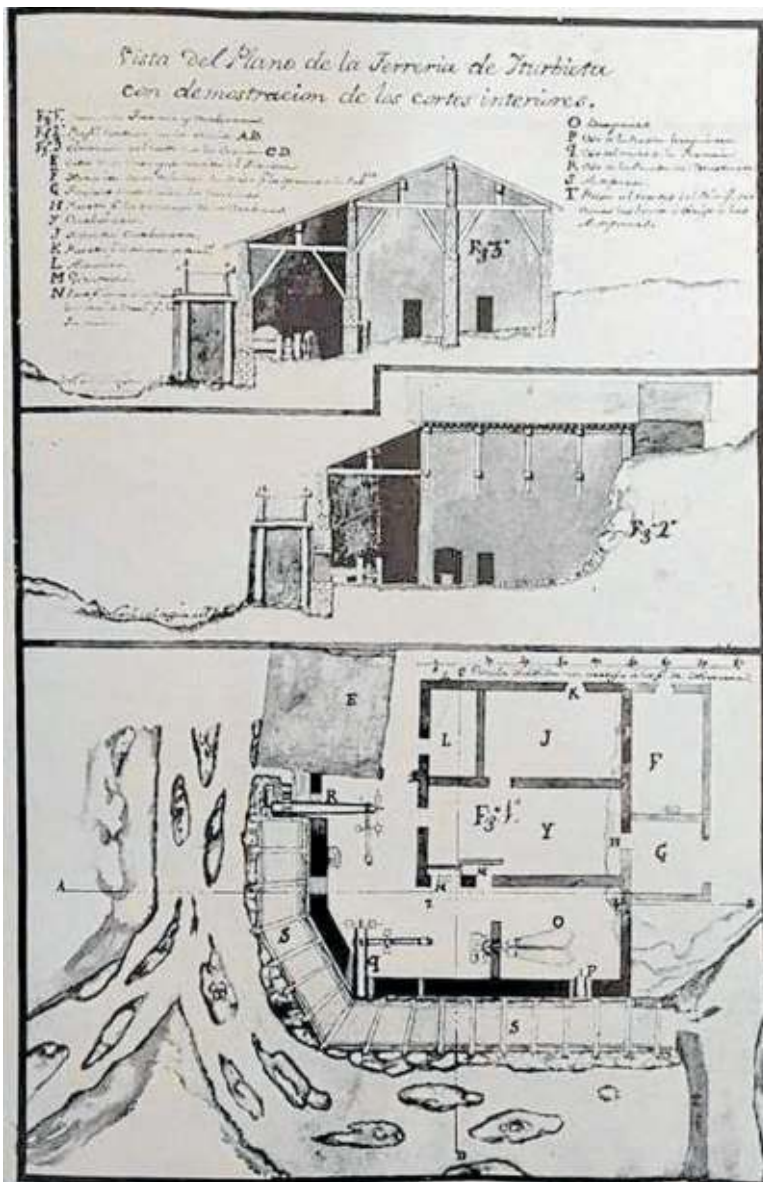
Zumarrezta edo Iturbia burdinolaren (Eratsun) oinplanta eta ebakidura 1801eko berreraikuntza planetan.
